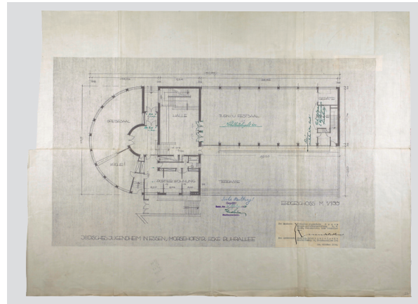
Abb. 6: Jüdisches Jugendheim in Essen, Grundriss Erdgeschoss, Genehmigungsplanung, datiert 20.10.1930. Stadtarchiv Essen, Bestand 143/1167.
