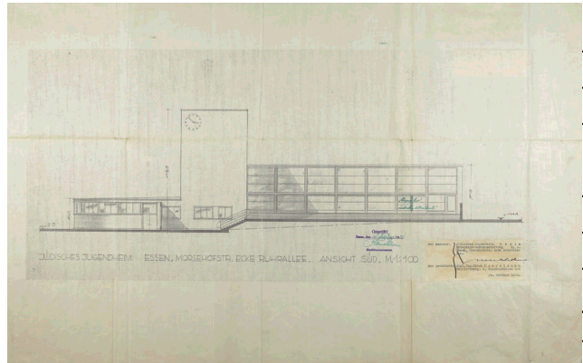
Abb. 8: Jüdisches Jugendheim in Essen, Ansicht Süd, Genehmigungsplanung, datiert 20.10.1930. Stadtarchiv Essen, Bestand 143/1167.
