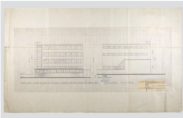
Abb. 7: Jüdisches Jugendheim in Essen, Ansichten West und Nord, Genehmigungsplanung, datiert 20.10.1930. Stadtarchiv Essen, Bestand 143/1167.
